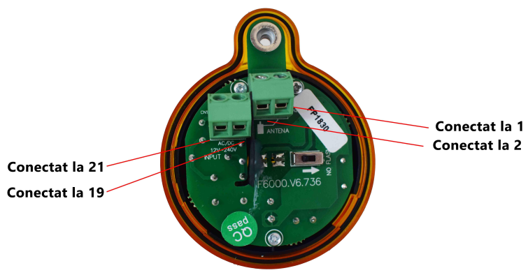
Schema conectare lampa de avertizare Lino (vezi schema de mai sus pentru referinta)
