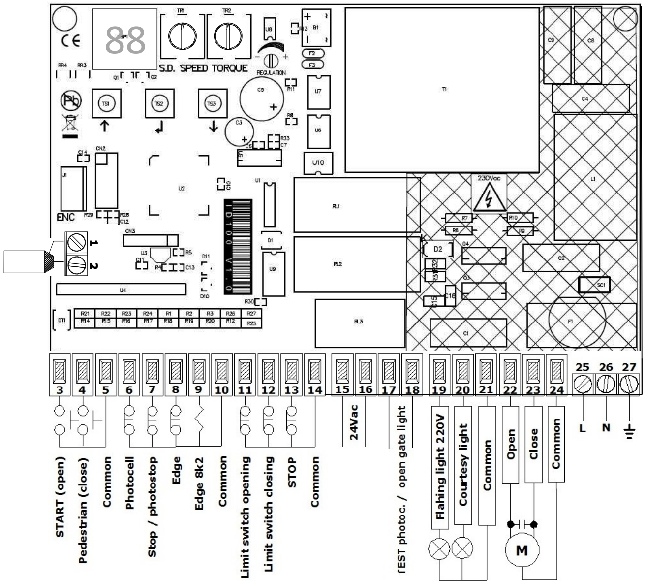
Schema conectare lampa de avertizare Lino (vezi schema de mai sus pentru referinta)
