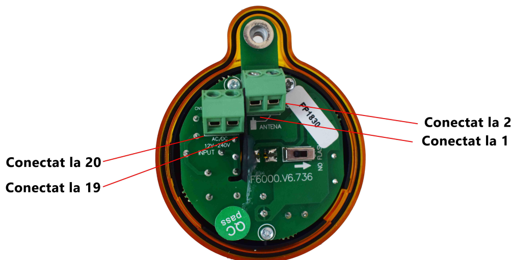
Schema conectare lampa de avertizare Lino (vezi schema de mai sus pentru referinta)
