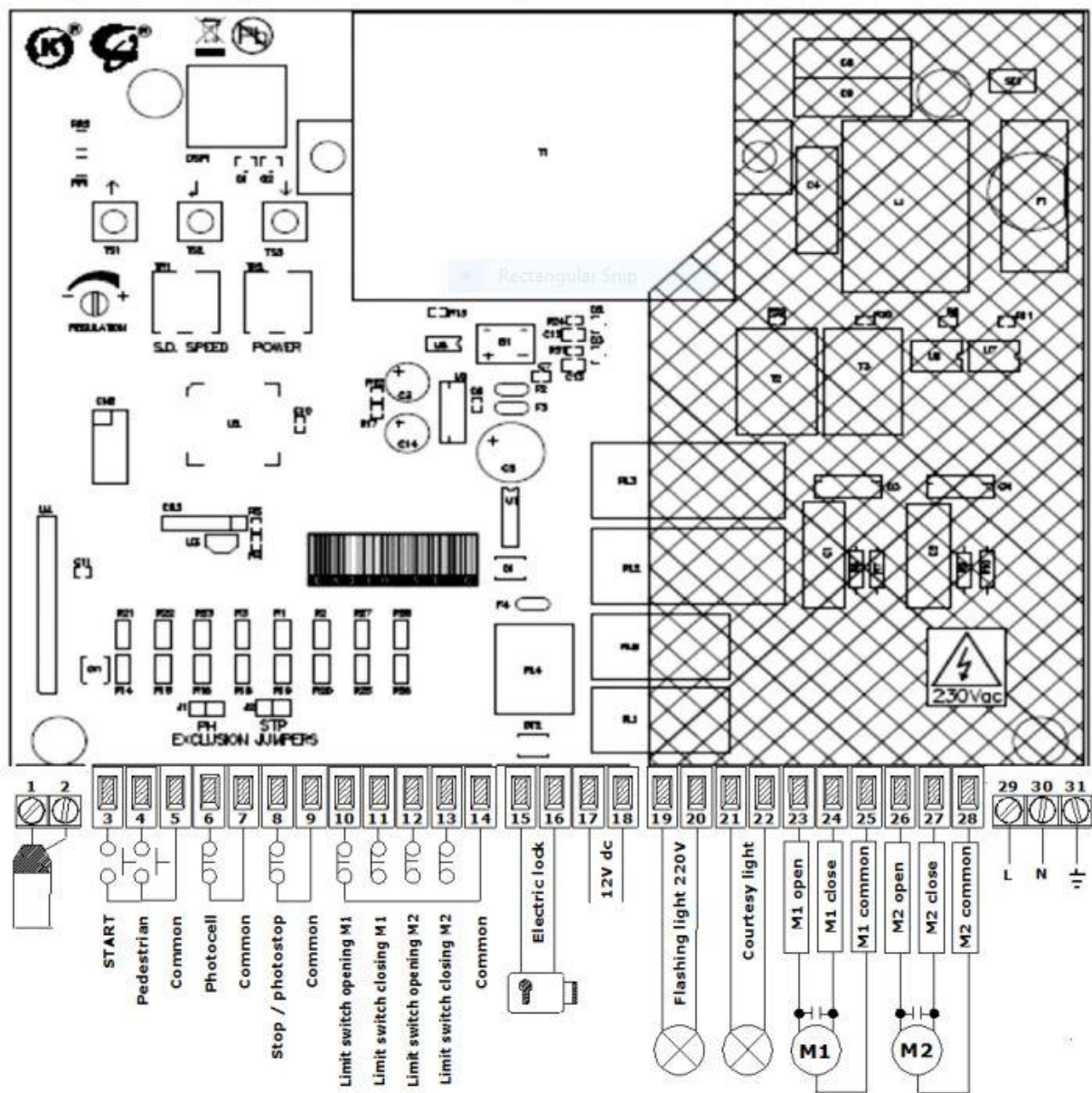
Schema conectare lampa de avertizare Lino (vezi schema de mai sus pentru referinta)
