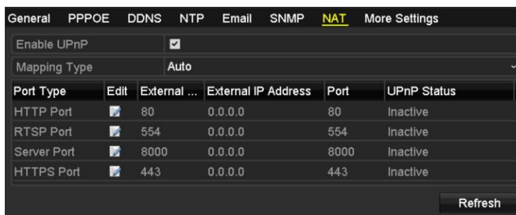
Figura 9. 17 Interfață Setări UPnP™
