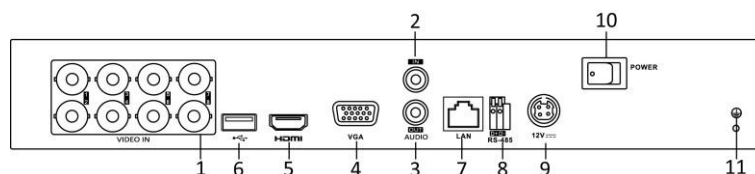
Figura 1. 11
