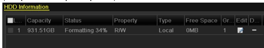
Figura 10.3 Inițializare Pornire
