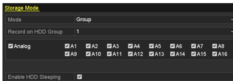
Figura 5. 28 HDD - Avansat
