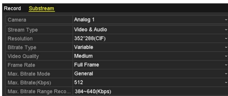
Figura 5. 5 Codificare sub-flux
