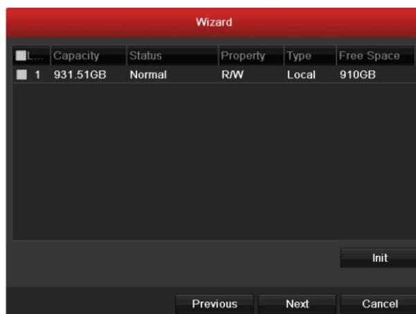
Figura 2. 9 Gestionare HDD
