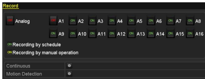
Figura 5.21 Înregistrare manuală
