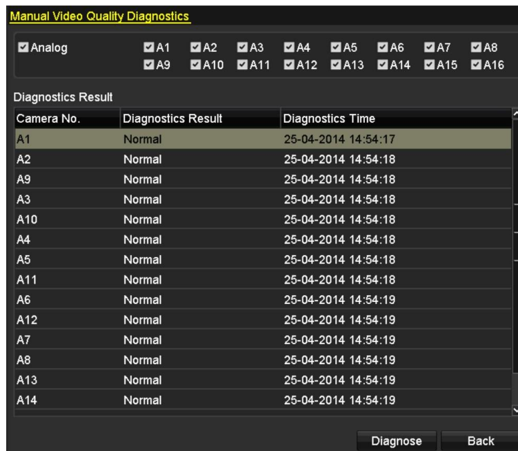
Figura 3. 11 Rezultat diagnosticare
