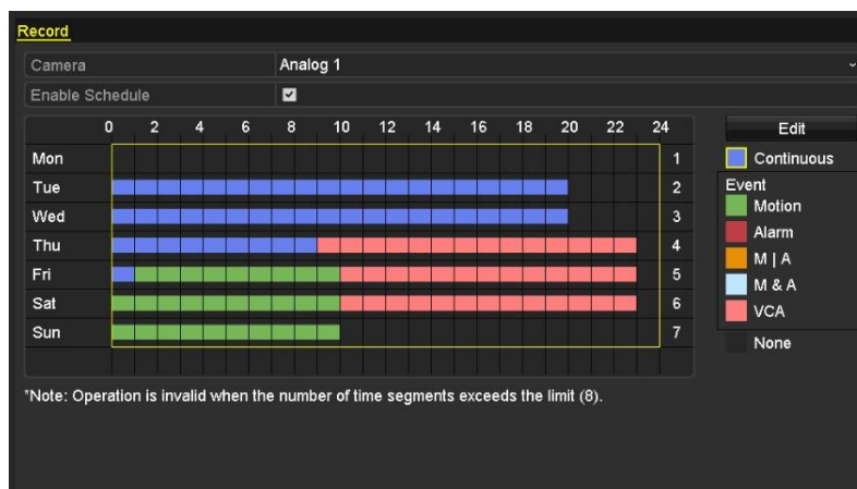
Figura 5. 10 Desenare program
