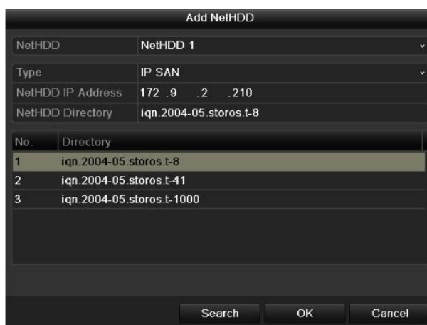
Figura 10. 9 Adăugare disk IP SAN
