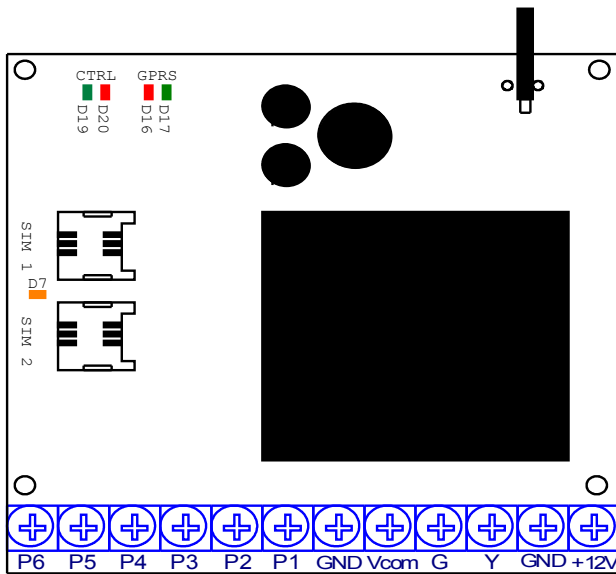
Figura 1: Diagrama modului
